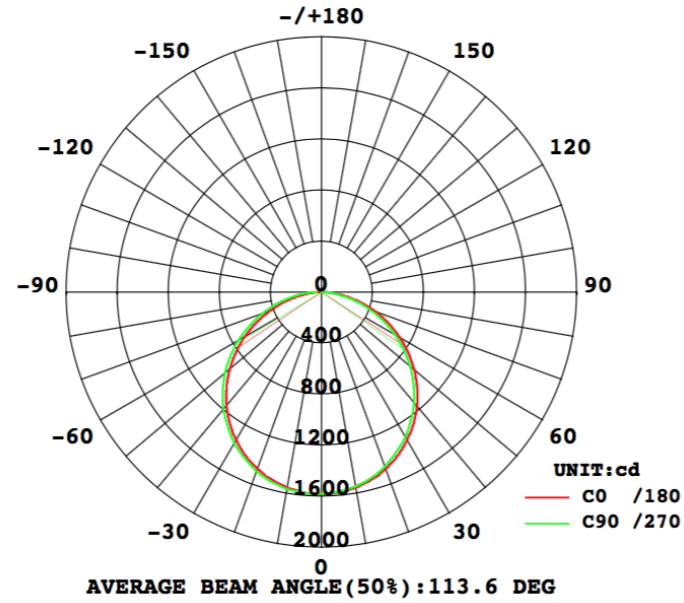
LLHT27-S048
